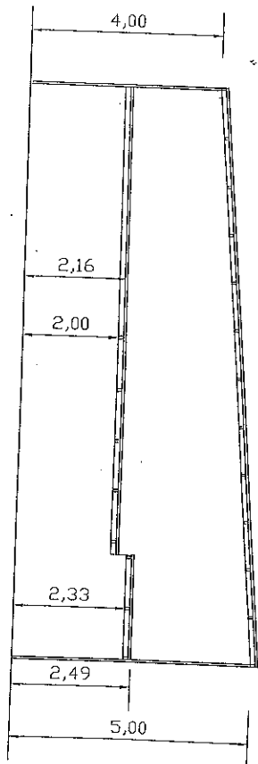
SEZIONE A-A
