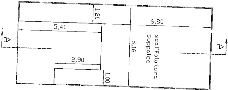
PIANO AMMEZZATO
